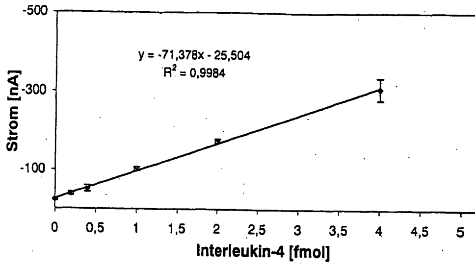
Abbildung 21: Kalibriergerade von Interleukin-4
